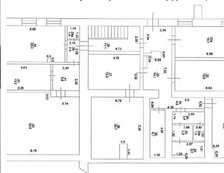
План 1 этажа (помещения 2Н площадью 242,3 кв.м.)
