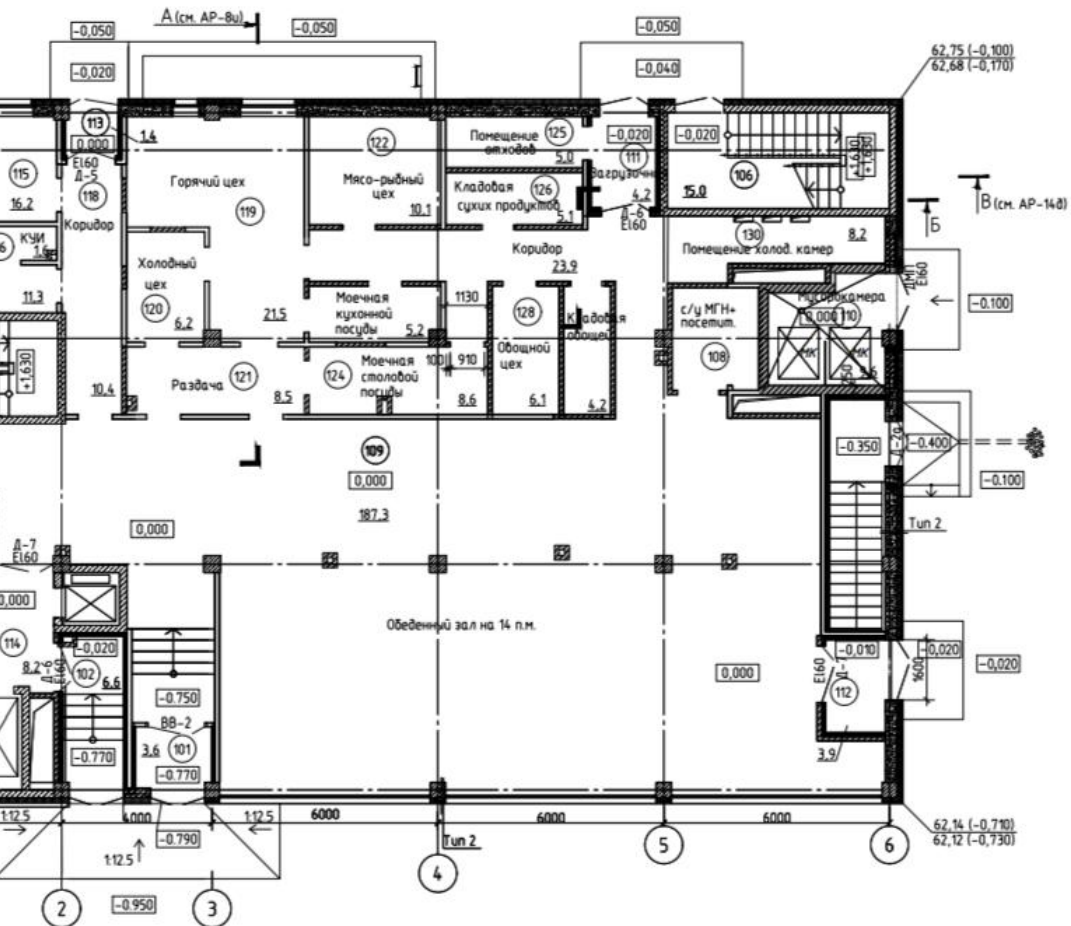
План первого этажа на отм.0.000 (1:100)
