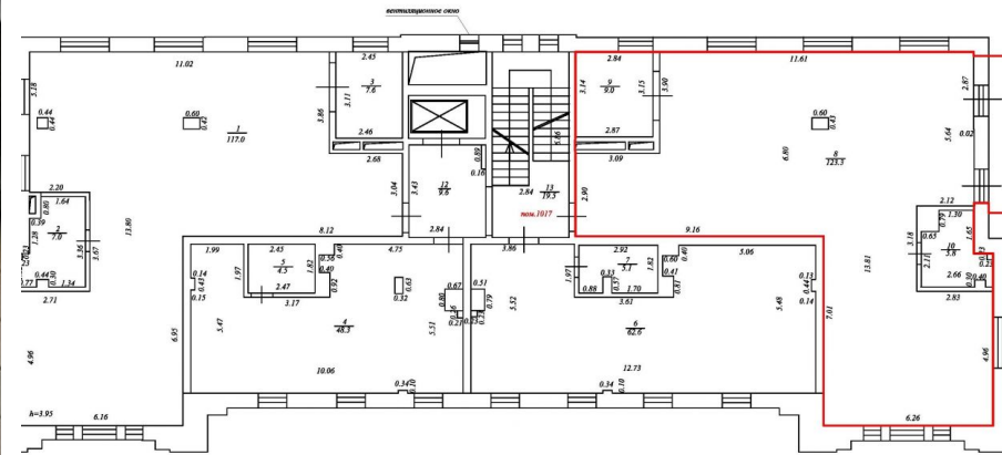
план 4 этажа
